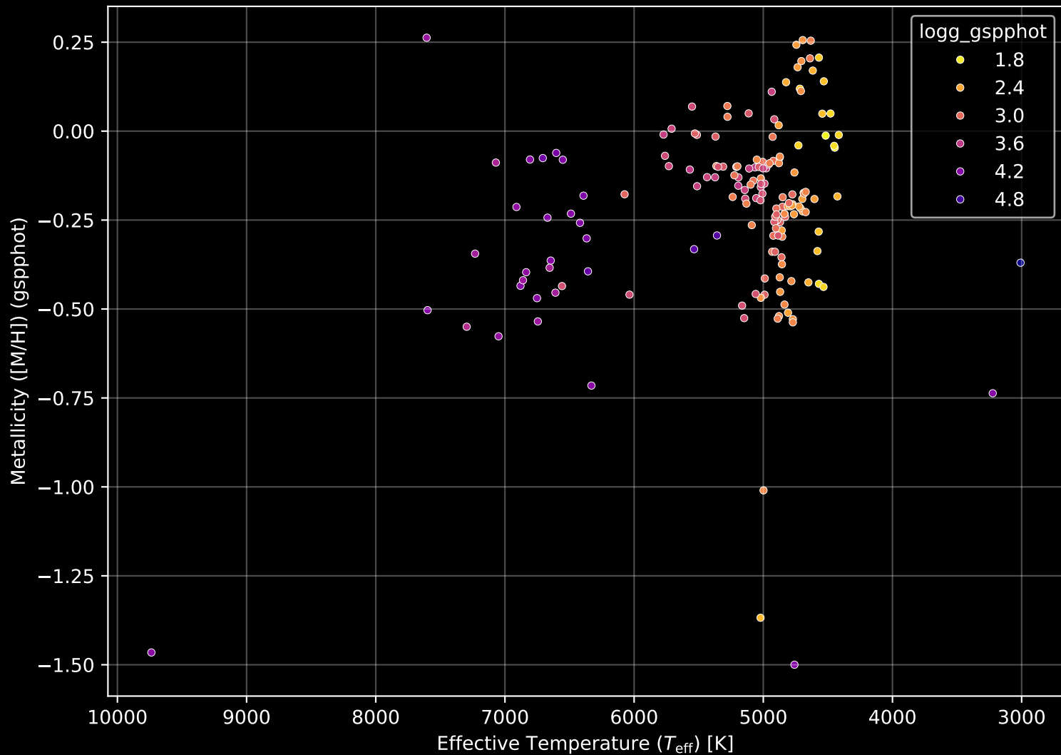
APOGEE DR17 Field: [210+30] Stellar Population Parameters (n= 172)
